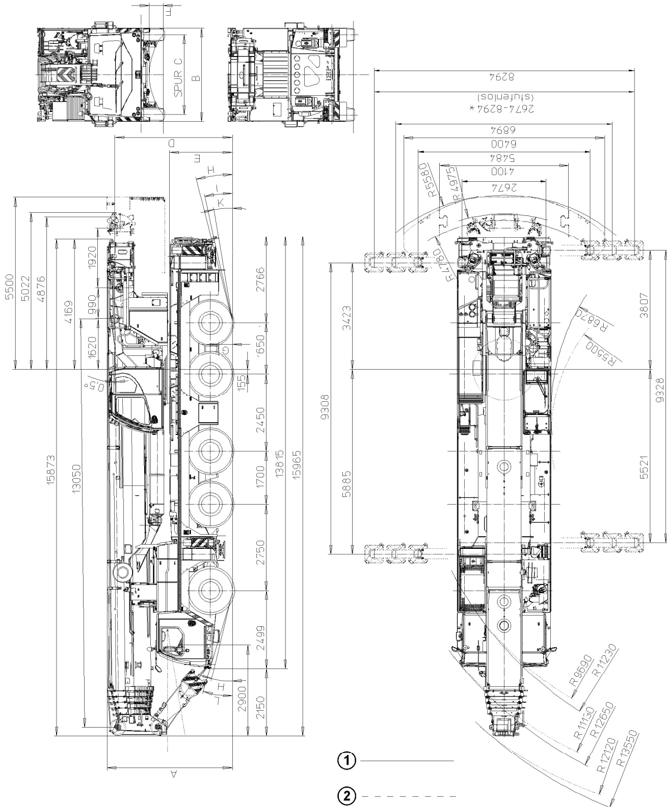
Fig.127962: Dimensiones
